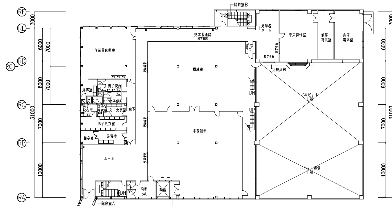
3階 平面図
